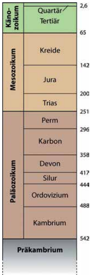
Abb. 4 Geologische Zeitskala, schematisch nach GTS2004 (GRADSTEIN et al. 2004). Zahlenwerte: Millionen [radiometrische] Jahre; Grafik aus JUNKER & SCHERER (2013).
