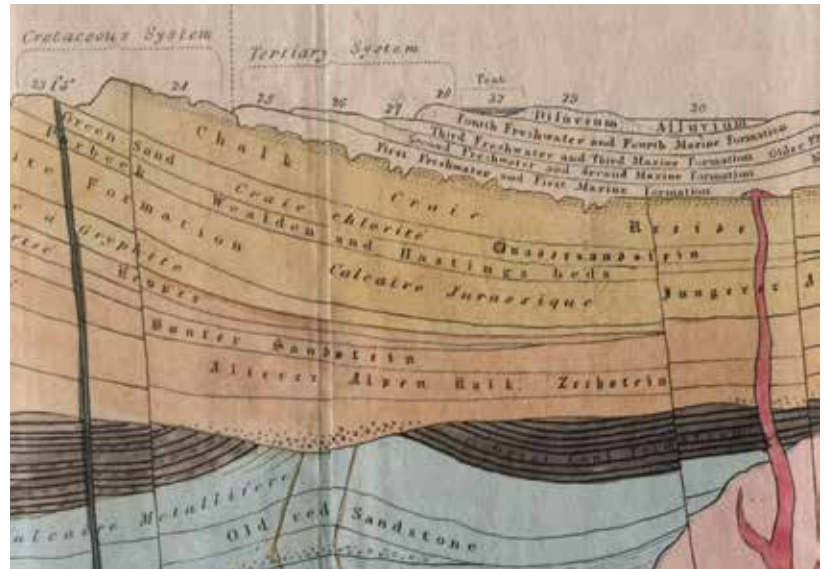
Abb. 5 William BUCKLANDs schematisches geologisches Profil von den Britischen Inseln bis zum Mittelmeer. Ausschnitt aus der etwa 1 m langen, gefalteten Tafel 1 (BUCKLAND 1838) mit stratigraphischen Einheiten vom Devon (Old Red Sandstone) bis zum Quartär (Diluvium, Alluvium).
