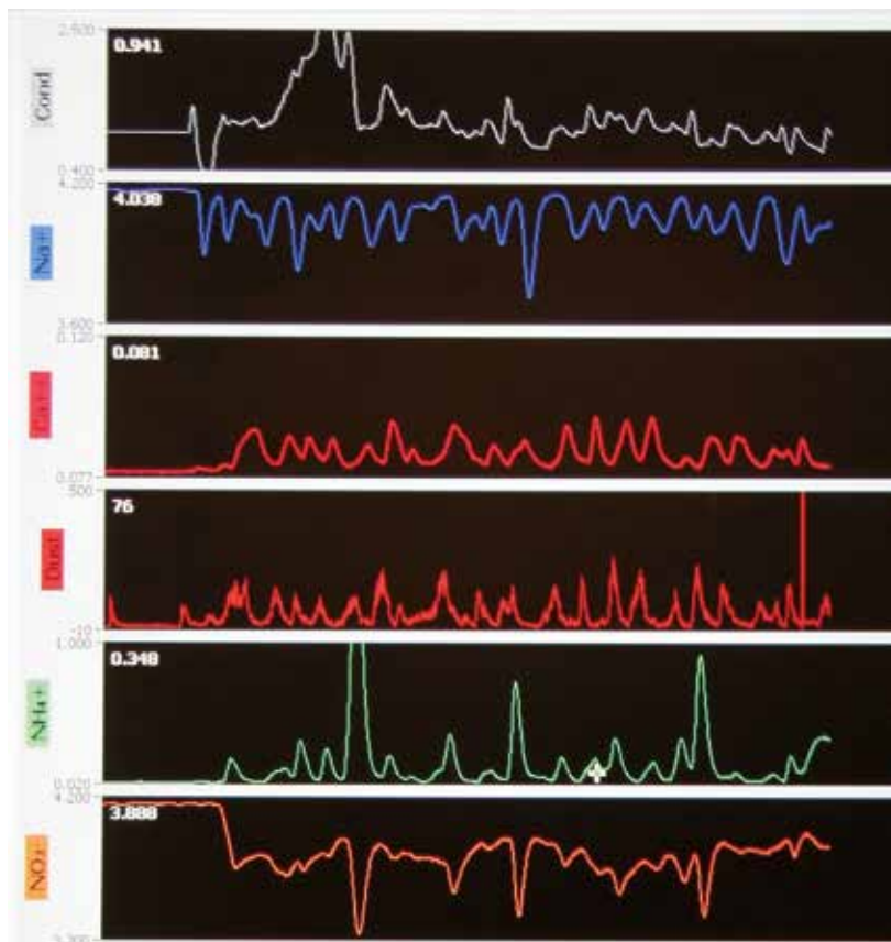
Abb. 5 Eiskernschmelzwasser-Reihenmessungen von Spurenstoffen, u. a. \text{NH}_4^+ , \text{Ca}^{2+} , \text{NO}_3^- , \text{Na}^+ , und Staub sowie der elektolytischen Leitfähigkeit mit CFA-Systemen (Continuous Flow Analysis). (Foto: Marie Kjaergaard; NEEM ice core drilling project, http://www.neem.ku.dk )
